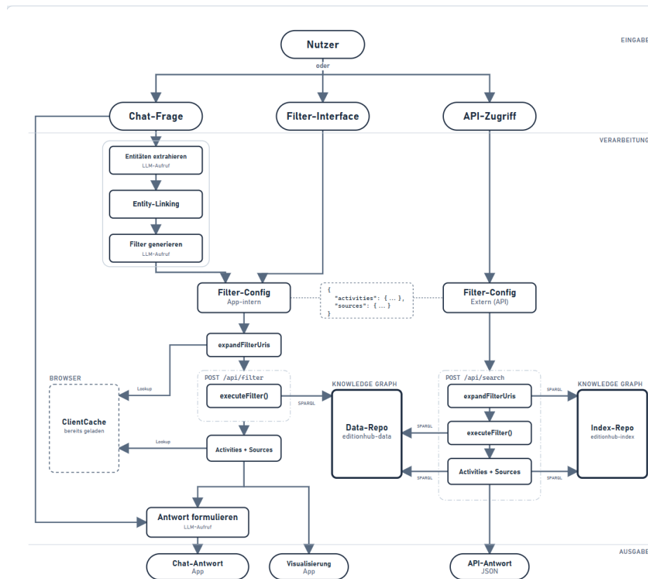
Abb.: Übersicht der drei Zugänge (API, Filter-Interface, KI-Chat) zum gemeinsamen Wissensgraphen.
