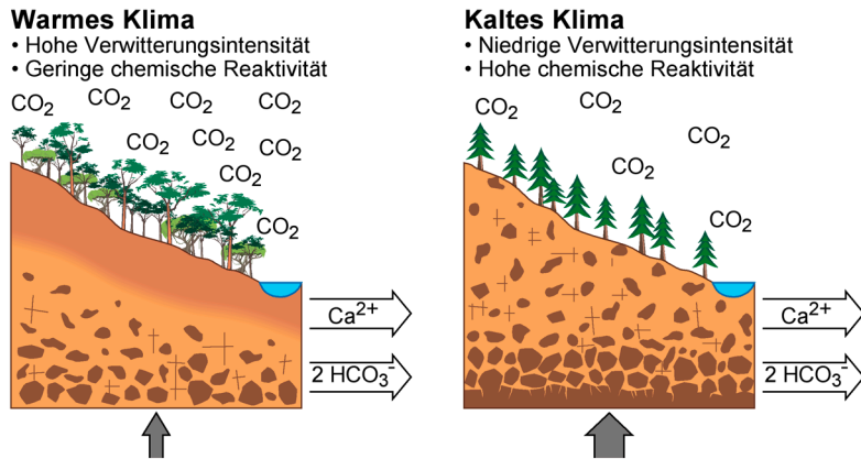
Abb. 5: Die „Reaktivität“ der Landoberfläche. Befinden sich mehr unverwitterte silikatische Mineralkörner wie Feldspat oder Glimmer im Boden, kann dieser mit wenig \text{CO}_2 ebenso gut chemisch reagieren wie ein bereits stark verwitterter Boden mit viel \text{CO}_2 ; die Verwitterungsrate (z. B. von \text{Ca}^{2+} ) und somit die Menge an \text{CO}_2 , die der Atmosphäre pro Zeitintervall entzogen wird, bleibt jedoch gleichförmig. (Quelle: F. von Blanckenburg, GFZ Potsdam, CC-BY 4.0)
