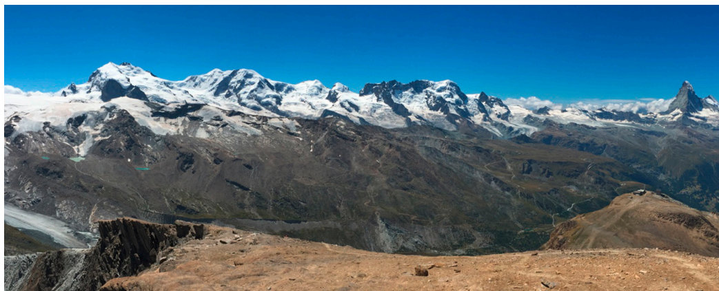
Abb. 4: Gebirgsbildung. Die Westalpen in Zermatt (Foto: F. von Blanckenburg, GFZ Potsdam)
