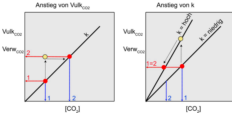
Abb. 3: Die mathematische Darstellung des Feedbacks zeigt, wie eine bestimmte vulkanische Emission \text{Vulk}_{\text{CO}_2} durch die Verwitterungs-Reaktionskonstante k die atmosphärische \text{CO}_2 -Konzentration [\text{CO}_2] bestimmt. Sind \text{Vulk}_{\text{CO}_2} und der \text{CO}_2 -Entzug durch Verwitterung \text{Verw}_{\text{CO}_2} balanciert, sind beide Größen auf der Y-Achse identisch. Links sehen wir einen Anstieg von \text{Vulk}_{\text{CO}_2} (1 auf 2). Vorübergehend ist der Kreislauf aus der Balance (gelber Kreis). Die Verwitterung holt aber auf, und das System ist wieder im Gleichgewicht (Position 2), allerdings bei höherem [\text{CO}_2] . Rechts sehen wir, was passiert, wenn die Reaktionskonstante k ansteigt, durch erhöhte Gebirgserosion z. B. Dann ist \text{Verw}_{\text{CO}_2} vorübergehend höher als \text{Vulk}_{\text{CO}_2} (gelber Kreis). Doch die Balance wird auch hier wieder hergestellt, weil [\text{CO}_2] fällt, so dass zum Schluss die gleiche Verwitterungsrate wie vorher herrscht, allerdings bei niedrigerem [\text{CO}_2] .
